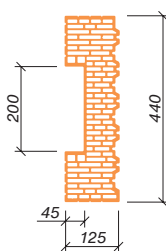
Porotherm 44 EKO+ Profi Dryfix 1/2 K (1/2 K = polovičná koncová)
