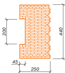
Porotherm 44 EKO+ Profi Dryfix K (K = koncová)
